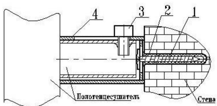
Сборка полотенцесушителя.
